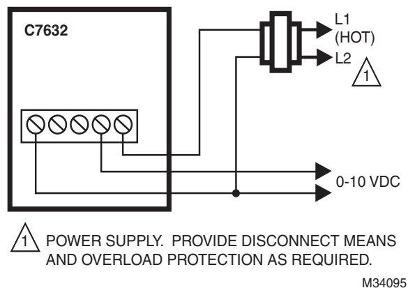
Fig. 3. Wiring for C7632
