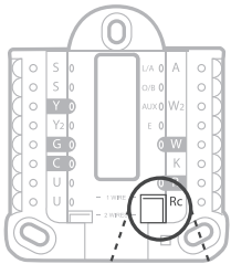
Système de montage UWP
